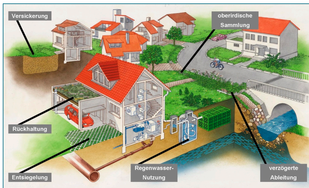
Abb. 3: Die wesentlichen Elemente der naturnahen Regenwasser- bewirtschaftung
